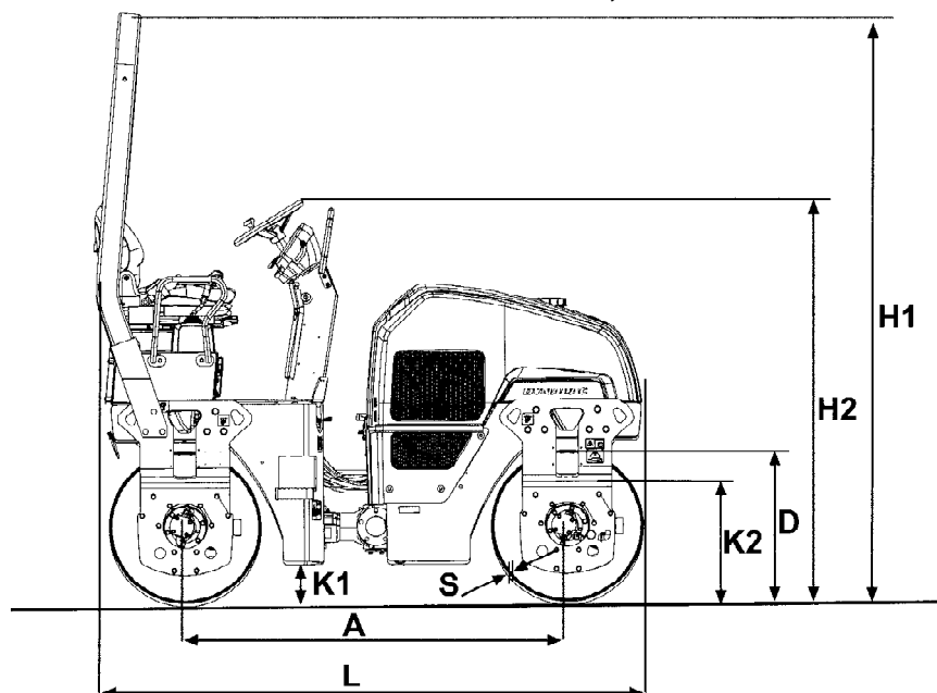
Dimensioni, vista laterale
