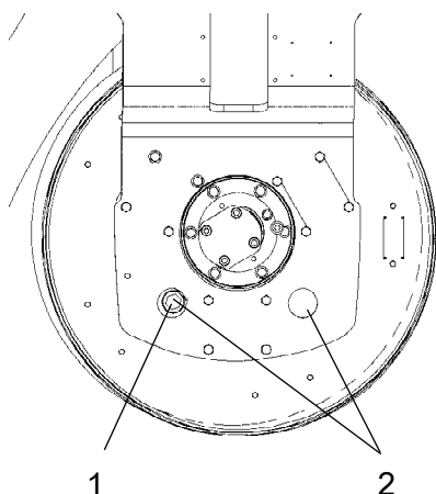
Fig. Tamburo, lato vibrazione 1. Tappo dell'olio 2. Foro d'ispezione
