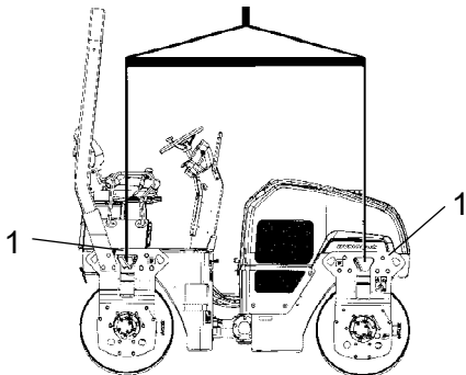
Fig. Sollevamento del rullo 1. Targhetta di sollevamento
