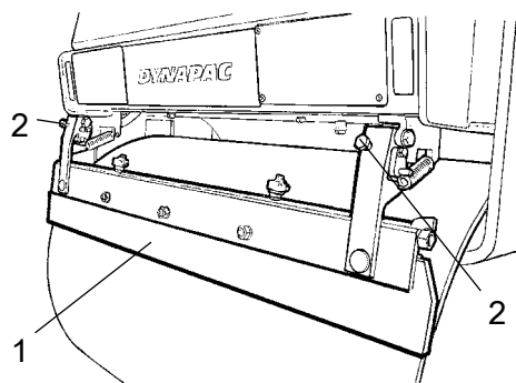
Fig. Raschietti elastici 1. Lama del raschietto 2. Viti di regolazione
