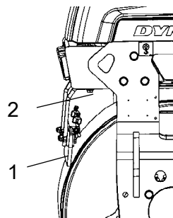
Fig. Taburo 1. Lama del raschietto 2. Viti di regolazione
