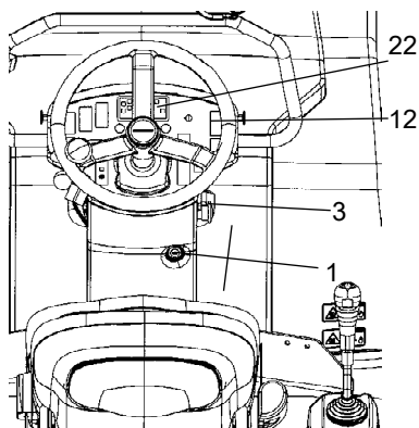
Fig. Pannello strumenti 1. Interruttore di avviamento 3. Arresto di emergenza 12. Interruttore irrorazione 22. Quadro delle spie
