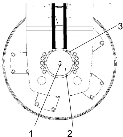
Fig. Lato sinistro del tamburo 1. Viti di rilascio 2. Alloggiamento del freno 3. Motore di trazione
