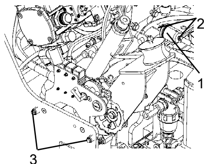
Fig. Vano motore 1. Prefiltro 2. Fascette stringitubo 3. Bulloni
