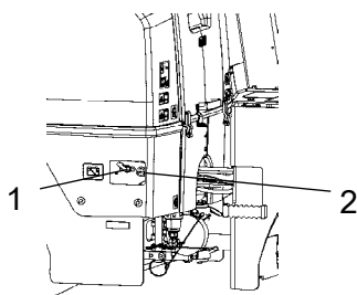
Fig. Vano batteria 1. Sezionatore batteria 2. Presa di alimentazione, 12 V
