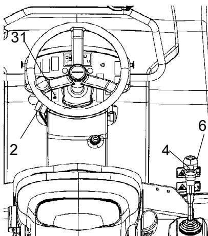
Fig. Quadro di comando 2. Comando dell'acceleratore 4. Vibrazione on/off 6. Leva di marcia avanti/indietro 31. Freno di parcheggio
