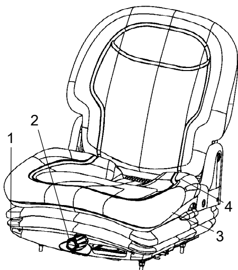
Fig. Sedile del conducente 1. Leva di bloccaggio - Regolazione in lunghezza 2. Regolazione del peso 3. Angolo di sostegno posteriore 4. Cintura di sicurezza
