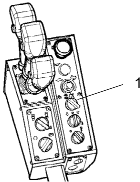
Fig. Tableau de bord 1. Commutateur, position transport/travail
