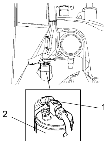
Fig. Filtre de séchage 1. Regard vitré 2. Porte-filtre
