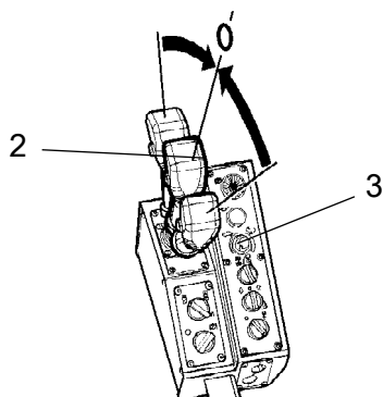
Fig. Tableau de bord 2. Commande de marche avant/arrière 3. Limitateur de vitesse
