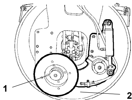
Fig. Disque/rouleau coupe-bordure 1. Position de transport 2. Position de fonctionnement
