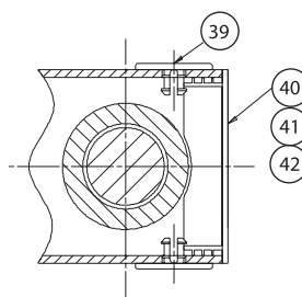
F - F
