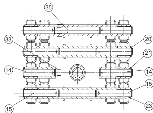
B - B
