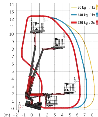
▶ Jibbi 1270 EVO
