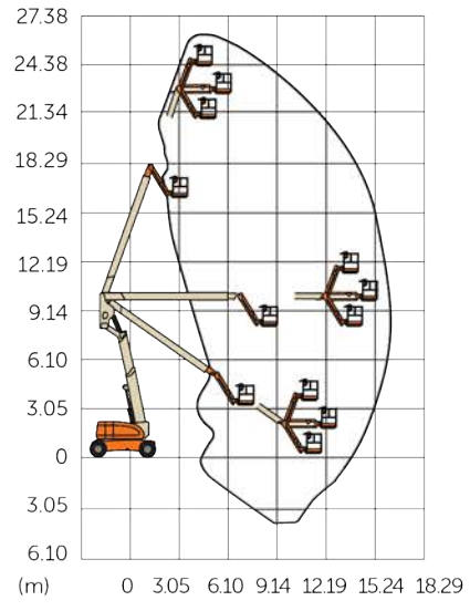
➤ JLG 800 AJ
