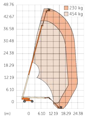
JLG 1500 SJ
