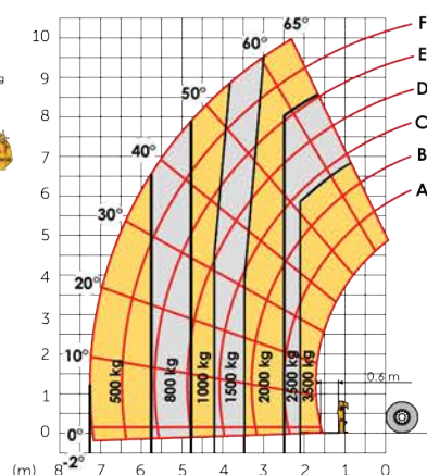
Haulotte HTL 3510
