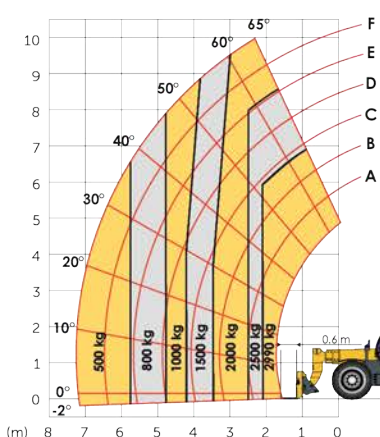
Haulotte HTL 3010
