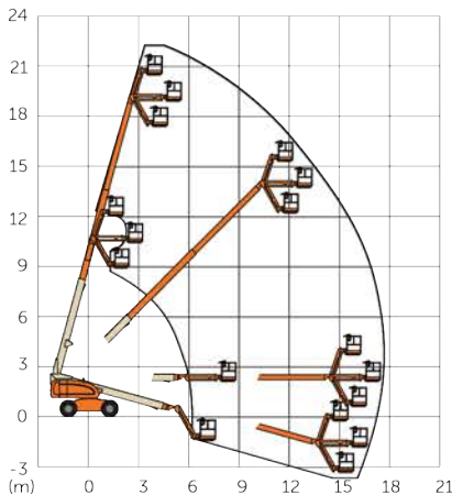
JLG 660 SJ
