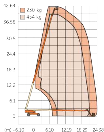
JLG 1350 SJP
