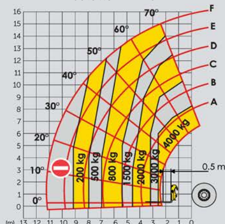
Haulotte HTL 4017
