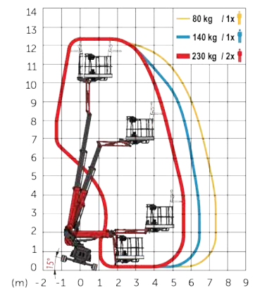
▶ Jibbi 1270 EVO
