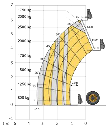
JCB 525-60
