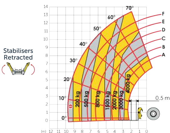
Haulotte HTL 4014
