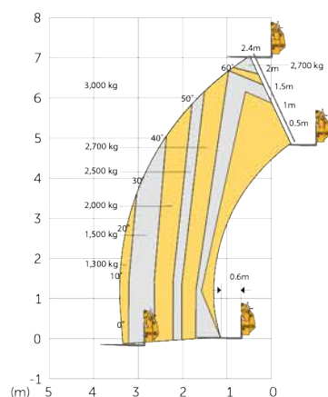
JCB 531-70
