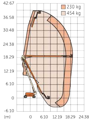
➤ JLG 1250 AJ
