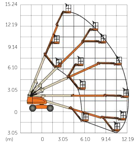
JLG 460 SJ
