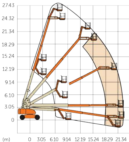
JLG 860 SJ
