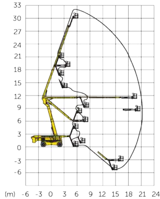
➤ JLG 1250 AJ
