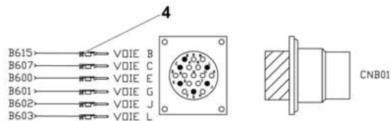
CONNECTEUR VUE INSERTION
