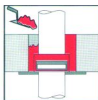
用CP636灰泥填充防火带周围的孔隙
