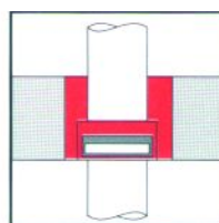
CP636固化后拆除模板
