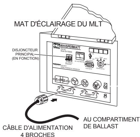
Figure 14. Disjoncteurs principal, GCFI (ON/MLT)
