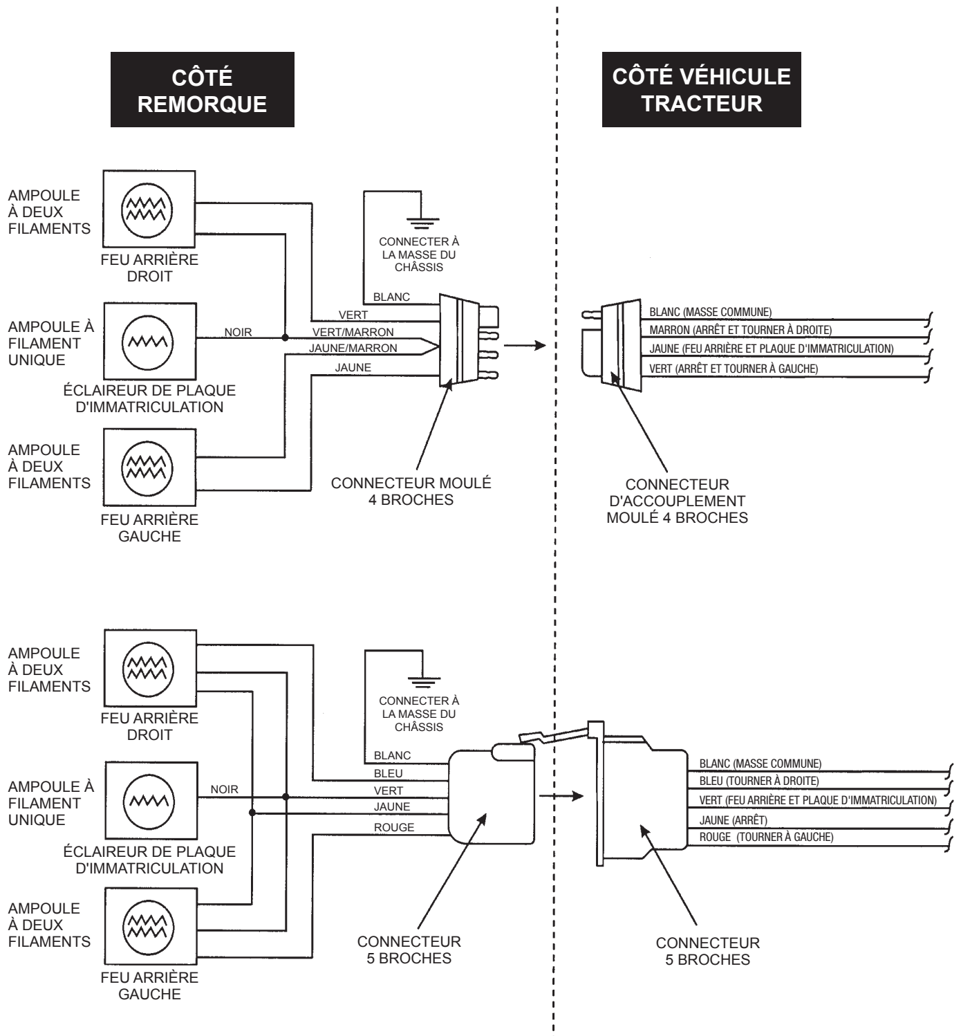
Figure 70. Schéma de câblage de la remorque/du véhicule tracteur
