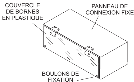
Figure 11. Couvercle en plastique (Cosses de sortie)
