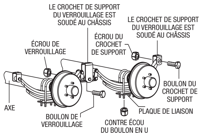
Figure 68. composants de la suspension à lames
