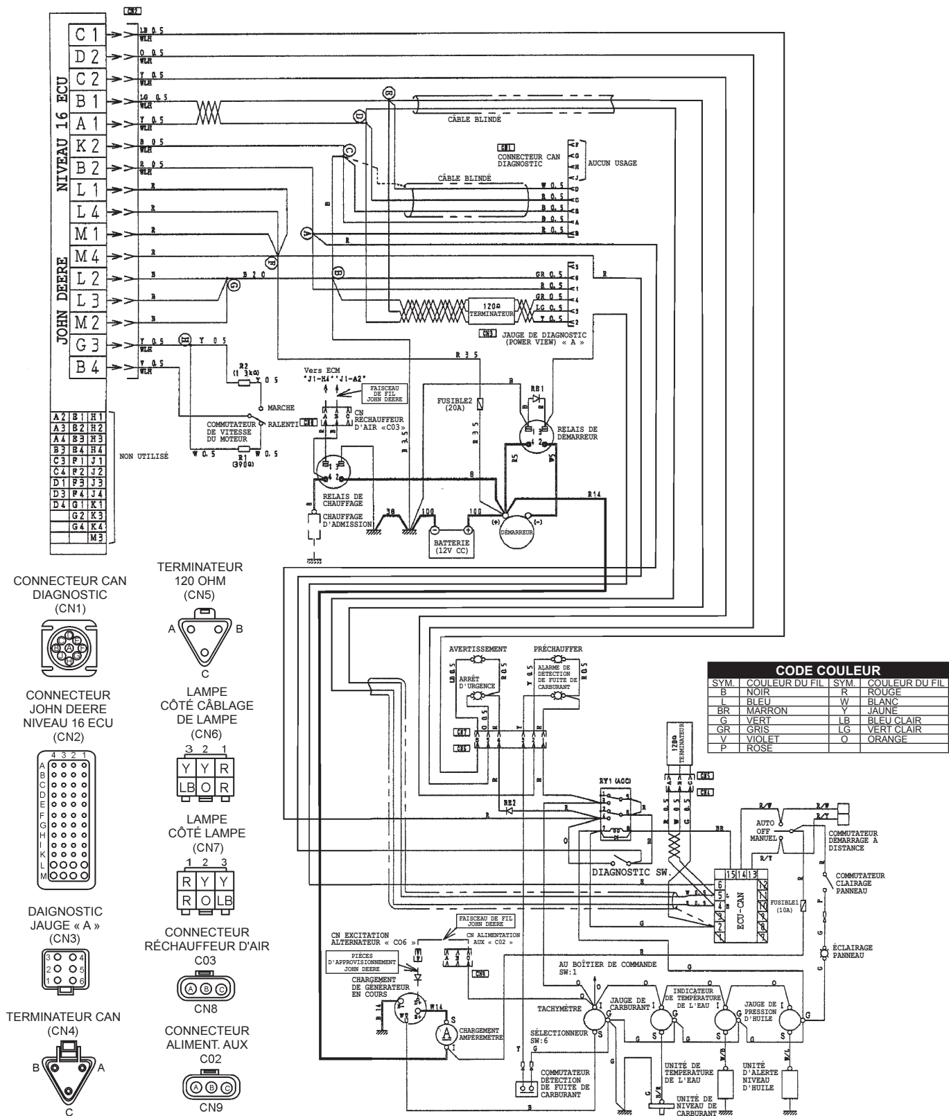
Figure 73. Schéma de câblage du moteur
