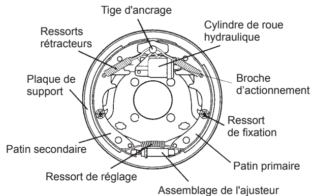
Figure 64. Composants du freinage hydraulique
