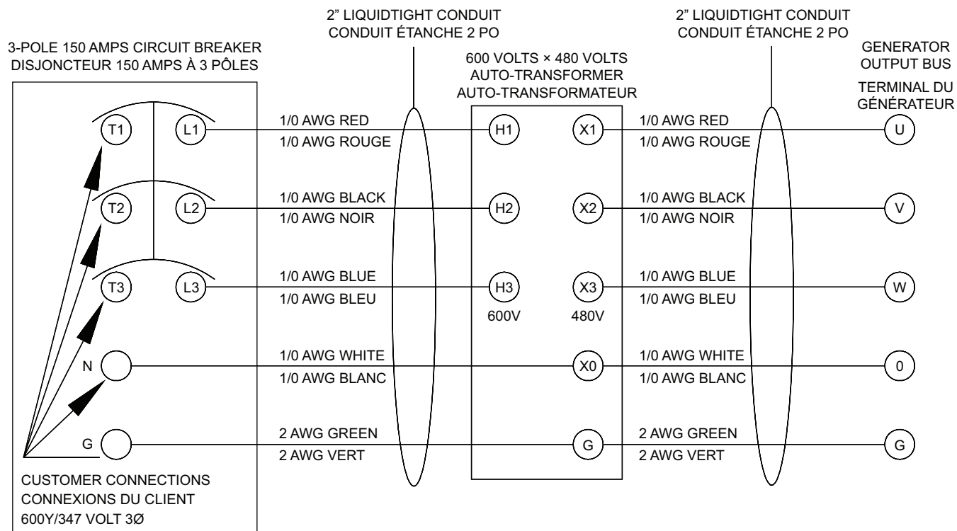
Figure 72. Schéma de câblage du transformateur automatique 3Ø
