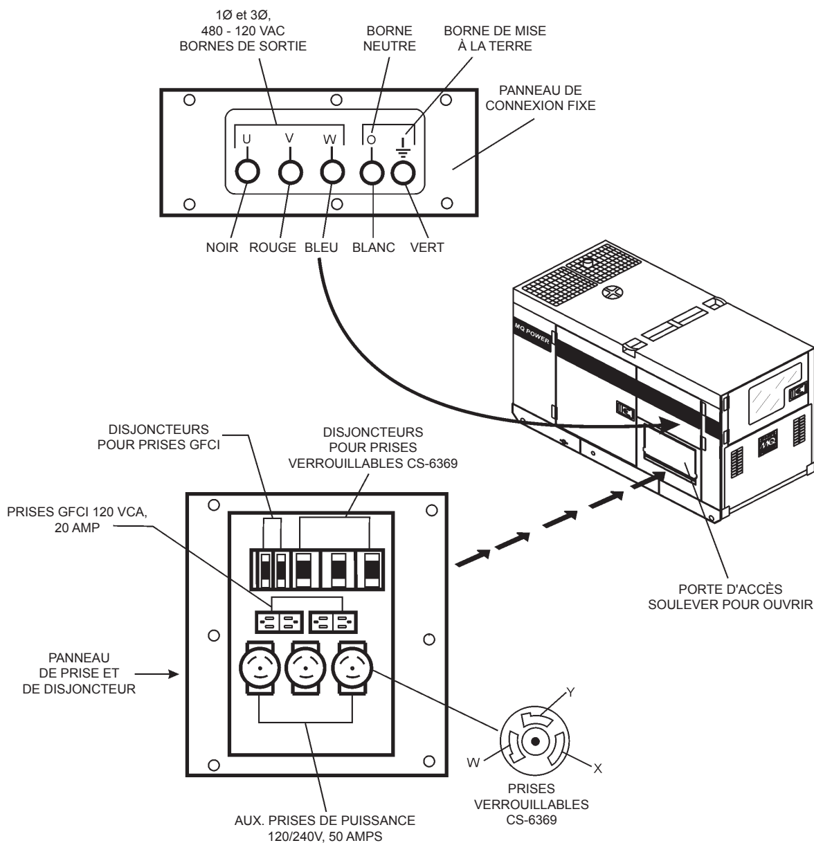
Figure 7. Panneau de bornes de sortie
