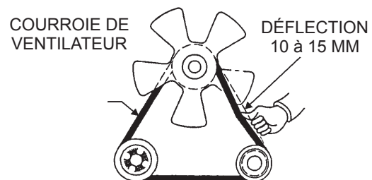
Figure 38. Tension de la courroie de ventilateur
