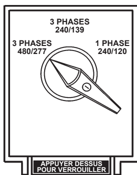
Figure 29. Commutateur de sélection de tension Position 3Ø-240/139V (transformateur automatique 600 V.c.a)
