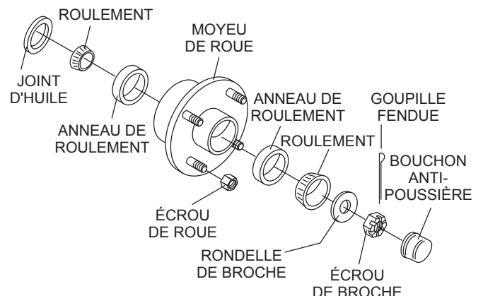
Figure 67. Composants du moyeu de roue
