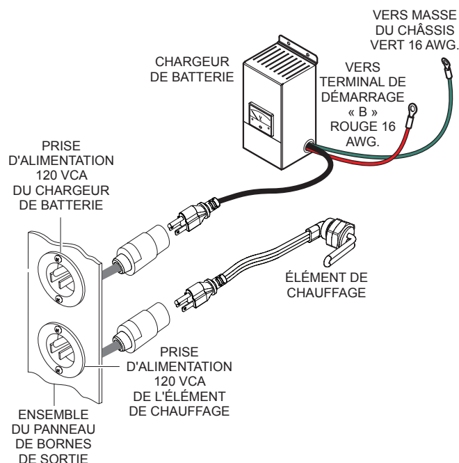
Figure 63. Connexions du chargeur de la batterie et de l'alimentation du chauffe-eau de l'enveloppe
