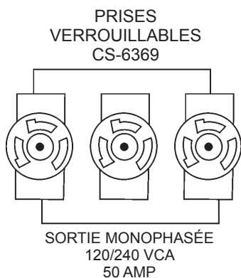
Figure 9. Prises auxiliaires verrouillables 120/240V
