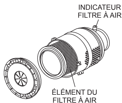
Figure 60. Filtre à air/indicateur
