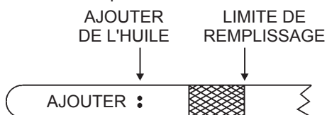
Figure 32. Jauge d'huile moteur
