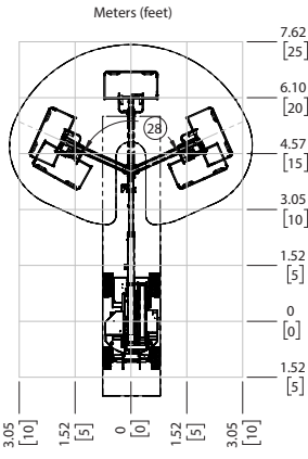
SJ45 ARJN ROTATING JIB
